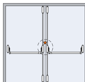
4-punts- vergrendeling met stompe deur
